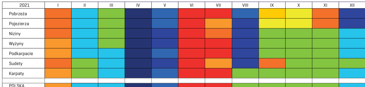
Wykres 2. Klasyfikacja warunków termicznych w poszczególnych miesiącach, według regionów w Polsce w 2021– dane IMGW
